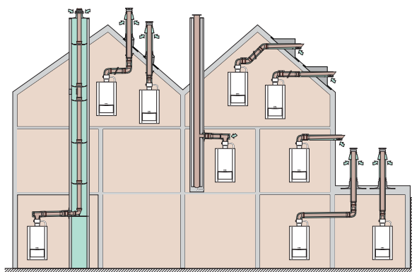
Možnosti různých instalací kondenzačních kotlů ecoTEC plus
