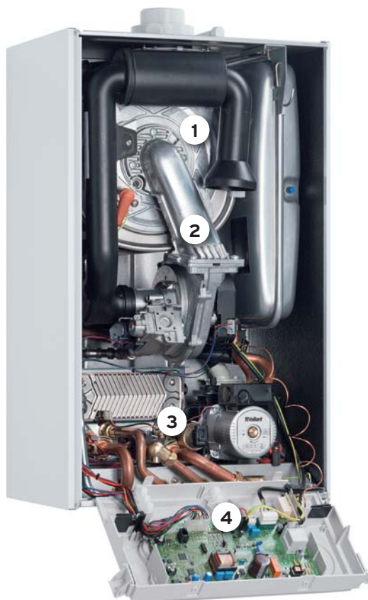
VUW 236/3-5 ecoTEC plus
